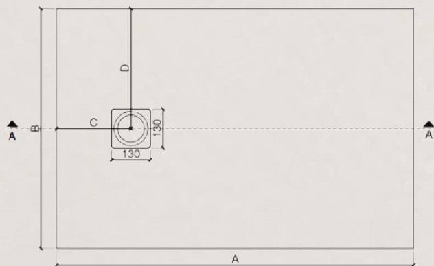
PIANTA
